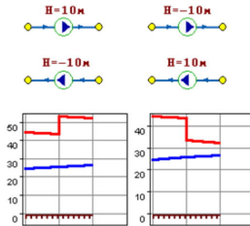
Рисунок 3.8 - Пьезометрические графики
